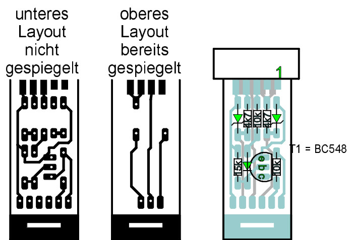
Serielles AVR-Programmer Interface Rev.3
